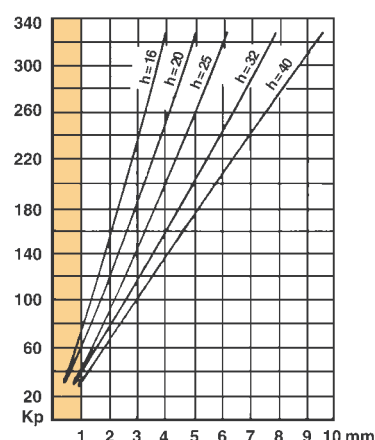
ø 20 - 95 SH 25% di compres. max
