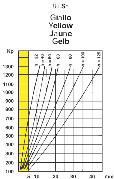
ø 63 - 80 SH 35% di compres. max
