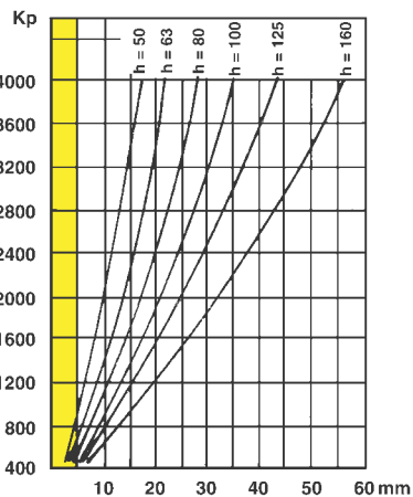
ø 100 - 80 SH 35% di compres. max
