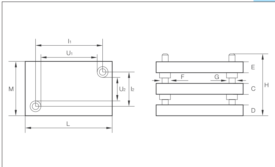
Dimensioni nominali mm / Nominal dimensions mm
